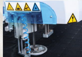
VORTEKS BIÇAK SOĞUTUCU VORTEX KNIFE COOLER Polyester ve bıçağa sıvama ihtimali olan kumaşlarda, soğutma sistemi ile engellenmesine olanak sağlar. Is Designed to Cool the knife with a Vortex Tube to reduce fusing with between plies when cutting difficult fabrics.
